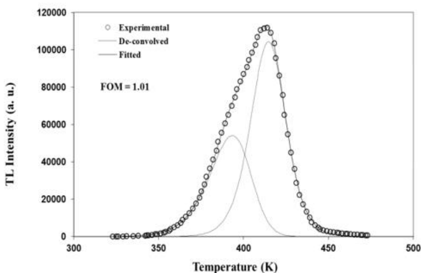
شکل ۹. منحنی برازش کامپیوتری بلور کلرید پتاسیم با ناخالصی دیسپرسیوم.
