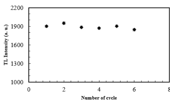
شکل ۱۰. منحنی درخشش ذرات KCl:Dy برای دزهای مختلف از ۱۰ تا ۱۰۰۰۰ Gy. شکل ۱۱. بررسی تکرارپذیری پاسخ ترمولومینسانس کلرید پتاسیم با ناخالصی دیسپرسیوم با دز ۱۰۰ Gy.
