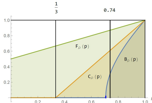
شکل ۱. (رنگی در نسخه الکترونیکی) نمودار پارامترهای نشانگر ناموضعییت B_\rho ، سنجهش درهم تنیدگی C_\rho و سنجهش فرابرد کوانتومی F_\rho بر حسب p برای حالت ورنر. دو خط عمودی \frac{1}{3} و 0.74 معادل حد بالای F_\rho برای فرابرد توسط به ترتیب کانال کلاسیکی و کانال سازگار با نظریه متغیر نهان موضعی هستند.
