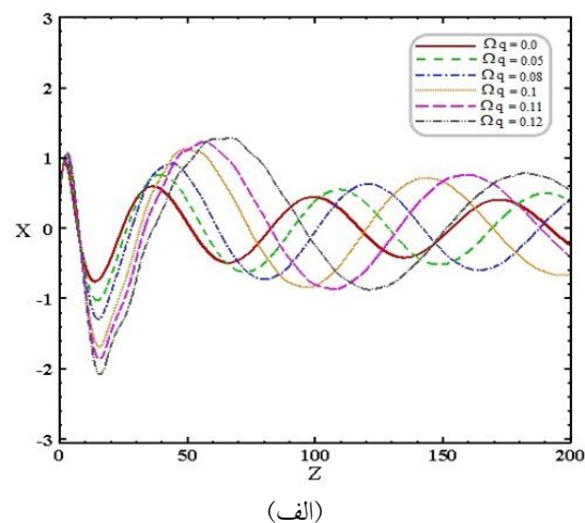
شکل ۱. (رنگی در نسخه الکترونیکی) مسیر حرکت الکترون بر حسب Z برای مقادیر متفاوت دامنه میدان ویگلری چهارقطبی (الف) در صفحه X-Z و (ب) در صفحه Y-Z .
