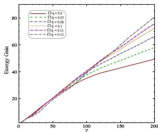
شکل ۲. (رنگی در نسخه الکترونیکی) انرژی الکترون بر حسب Z (رنگی در نسخه الکترونیکی) نمودار بیشینه انرژی الکترون برای حسب دامنه میدان ویگلری چهارقطبی.
