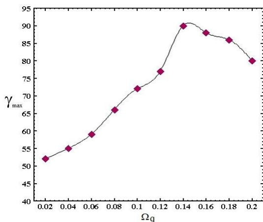
شکل ۳. (رنگی در نسخه الکترونیکی) نمودار بیشینه انرژی الکترون برای حسب دامنه میدان ویگلری چهارقطبی.
