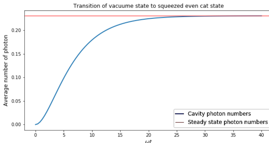
شکل ۶. (رنگی در نسخه الکترونیکی) مقادیر میانگین تعداد فوتون‌های کاواک \bar{n} = \langle a^\dagger a \rangle ، در تماس با یک محیط سرد با اتلاف دوفوتونی به صورت تابعی از زمان بهنجار شده \omega t . پس از حدود بیست و پنج واحد زمانی میانگین فوتون‌ها به مقدار تعادلی حدود 0.23 می‌رسد.
