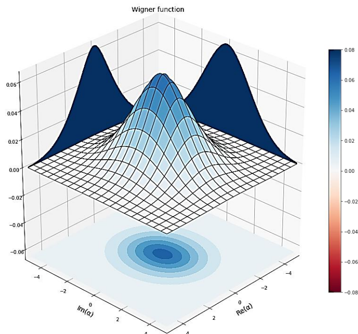
شکل ۱۷. تابع ویگنر تابش نهایی به صورت سه بعدی. قسمت حقیقی \alpha متناسب با X_1 و قسمت موهومی \alpha متناسب با X_2 است. گرمای محیط چلانگی را از بین برده است.
