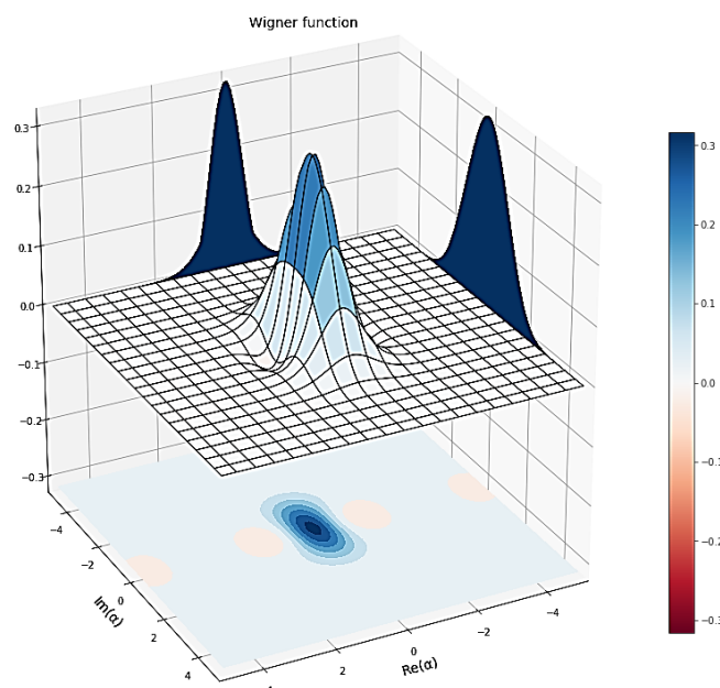
شکل ۱۱. (رنگی در نسخه الکترونیکی) تابع ویگنر تابش نهایی به صورت سه بعدی. قسمت حقیقی \alpha متناسب با X_1 و قسمت موهومی \alpha متناسب با X_2 است. چلانگی در X_1 از روی شکل مشخص است.
