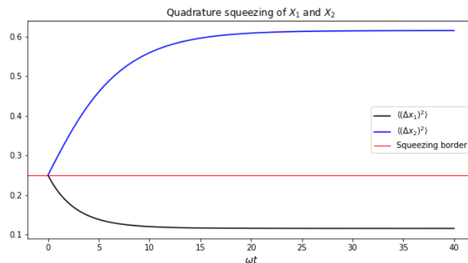
شکل ۷. (رنگی در نسخه الکترونیکی) واریانس دو عملگر تربیع به صورت تابعی از زمان بهنجار شده \omega t ، پس از تماس با یک منبع سرد با اتلاف دوفوتونی. خط قرمز مرز چلانگی را نشان می‌دهد.
