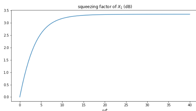
شکل ۸. (رنگی در نسخه الکترونیکی) عامل چلانگی عملگر تربیع \hat{X}_1 برحسب دسی‌بل، به صورت تابعی از زمان بهنجار شده \omega t پس از تماس با یک محیط سرد با اتلاف دوفوتونی.
