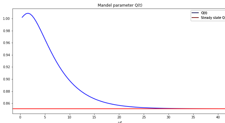
شکل ۱۲. (رنگی در نسخه الکترونیکی) پارامتر مندل برای تابش کاواک، به صورت تابعی از زمان بهنجار شده \omega t . خط قرمز همین پارامتر را پس از رسیدن به حالت تعادل نهایی نشان می‌دهد.
