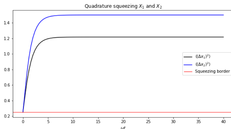
شکل ۱۵. (رنگی در نسخه الکترونیکی) واریانس دو عملگر تربیع به صورت تابعی از زمان بهنجار شده. خط قرمز مرز چلانگی را نشان می‌دهد. گرمای محیط چلانگی را کاملاً از بین برده است.
