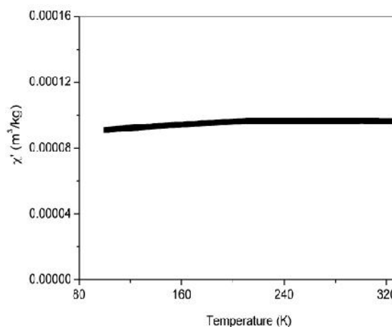
شکل ۴. پذیرفتاری مغناطیسی نمونه پس از ۲۰ ساعت آسیاب‌کاری.
