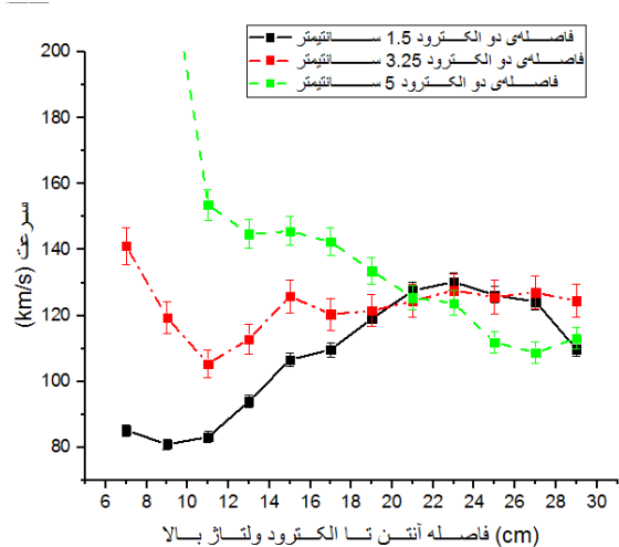
شکل ۹. نمودار تغییرات سرعت متوسط گلوله‌های پلاسمایی برای فاصله بین دو اکتروود ۱/۵ سانتی‌متر (خط سیاه)، ۳/۲۵ سانتی‌متر (خط نقطه چین قرمز) و ۵ سانتی‌متر (خط چین سبز).
