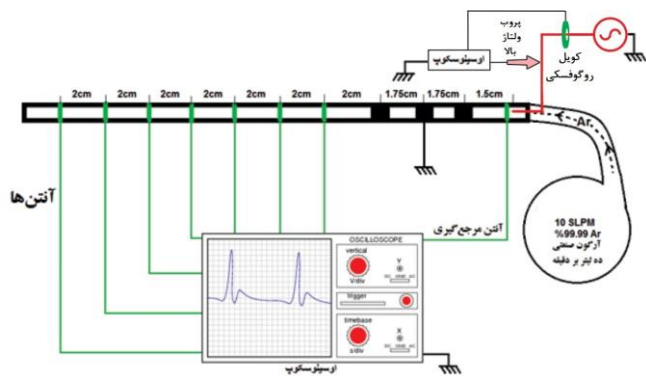
شکل ۶. پیکربندی و نحوه اتصال منبع تغذیه به فواره در تمام آزمایش‌ها. شکل ۷. طرحواره کلی چیدمان آزمایش.
