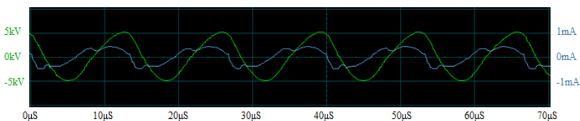
شکل ۸. نمایی از ولتاژ منبع تغذیه (در حالت بار) و گلوله آشکار شده در آنتن مرجع‌گیری. نمودار سبز رنگ مربوط به ولتاژ و نمودار آبی رنگ مربوط به جریان می‌باشد.
