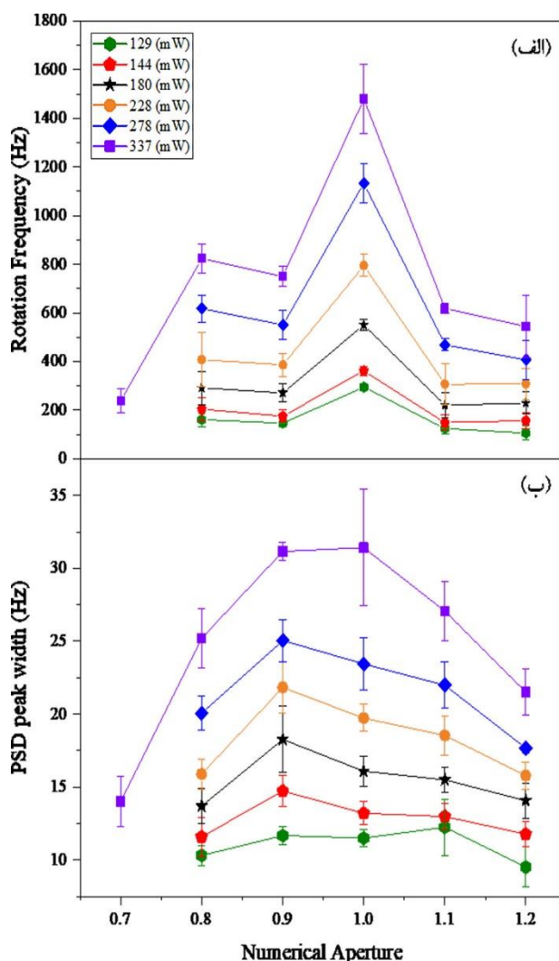
شکل ۴. نتایج اثر تغییر گشودگی عدسی بر روی (الف) بسامد چرخش و (ب) پهناي بسامدی قله چرخشی که با استفاده از روش طیف توانی به دست آمده است.
