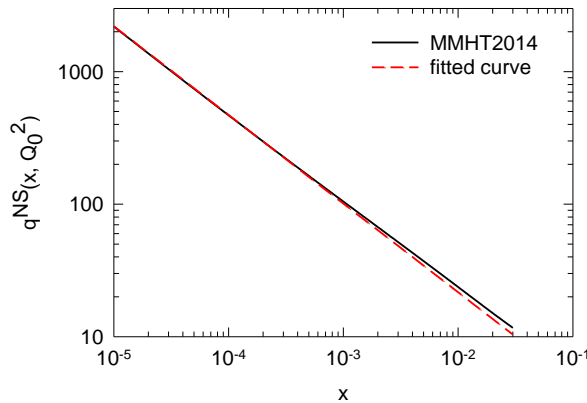
شکل ۲. نمودار برازش حل تحلیلی معادله DGLAP با تابع توزیع نایکتای کوارکی معمولی MMHT2014 در Q_0^2 = 1 \text{ GeV}^2 در بازه تغییرات x: [10^{-5}, 0/03] .
