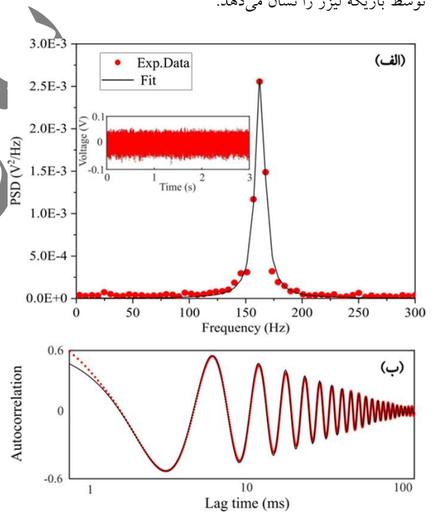
شکل ۲. (الف) نتایج تحلیل طیف توانی و (ب) نتایج تحلیل خود همبستگی از سیگنال فوتودیود برای یک نانوذره در حال چرخش در تله نوری (نقاط قرمز رنگ). نمودار پیوسته مشکی در (الف) برازش معادله (۲) به نتایج طیف توانی و در (ب) برازش معادله (۳) به نتایج خودهمبستگی را نشان می‌دهد. نمودار قرارداده شده در داخل قسمت (الف) ولتاژ افت و خیز حرکت ذره در حال چرخش را نشان می‌دهد که برحسب زمان رسم شده است.
