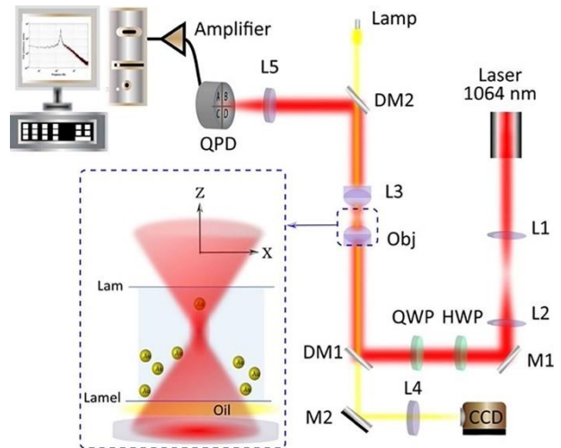
شکل ۱. طرح‌واره چیدمان آزمایشگاهی تله‌اندازی و چرخش ذرات. در این چیدمان L, M, DM, QWP, HWP, QPD و ترتیب عدسی، آینه، تیغه نیم‌موج، تیغه ربع‌موج و فوتودیود چهارتابی هستند. مربع خط چین تصویر بزرگ شده‌ای از داخل نمونه و تله‌اندازی ذرات توسط باریکه لیزر را نشان می‌دهد.
