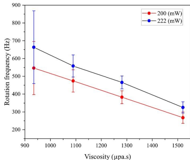
شکل ۶. اثر شکسانی محیط بر روی سرعت چرخش ذره. فرکانس چرخش بر حسب شکسانی مخلوط آب و گلیسرین با نسبت‌های مختلف، برای دو توان لیزر مختلف ۲۰۰ mW و ۲۲۲ mW قبل از عدسی شیئی رسم شده است.
