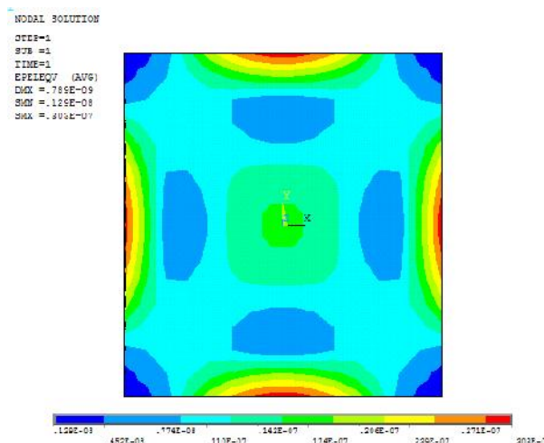
شکل ۴. (رنگی در نسخه الکترونیکی) کرنش فون میزس دريچه مربعی به ضلع ۳ mm وضخامت ۲۰ μm با اعمال فشار یکنواخت یک پاسکال.
