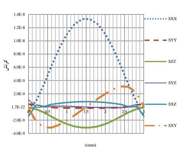
شکل ۳. (رنگی در نسخه الکترونیکی) کرنش در عمق ۵ میکرومتری در محل موج‌بر (با فاصله ۱۰۰ میکرومتر از لبه دريچه) بر اثر اعمال فشار یکنواخت یک پاسکال.
