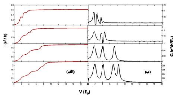
شکل ۲. (الف) نمودار جریان برحسب ولتاژ در چهار حالت از ترکیب چهار نقطه کوانتومی. (ب) نمودار هدایت برحسب ولتاژ در چهار حالت از ترکیب چهار نقطه کوانتومی جفت شده به الکترودهای فلزی.
