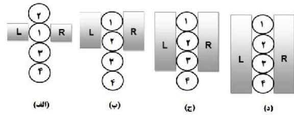
شکل ۱. چهار حالت از ترکیبات چهار نقطه کوانتومی جفت شده به الکتروودهای فلزی در دمای صفر.
