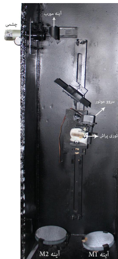
شکل ۱۲. (رنگی در نسخه الکترونیکی) نمایی از دو آینه و توری پراش.
