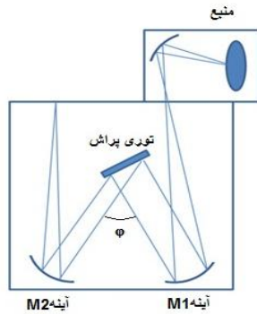
شکل ۱۰. مونوکروماتور [۷].
