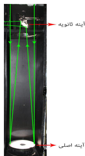
شکل ۶. (رنگی در نسخه الکترونیکی) مسیر حرکت نور در تلسکوپ.
