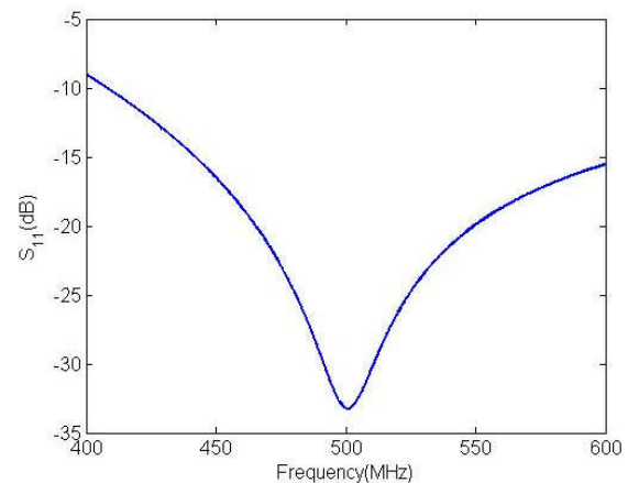
شکل ۶. نمودار تلف بازگشتی S_{11} بر حسب بسامد.
