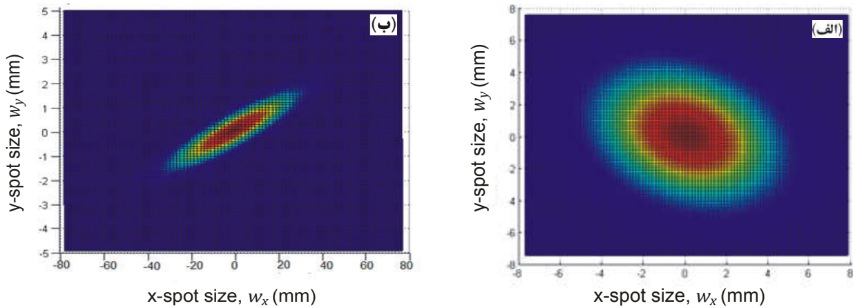
شکل ۹. (رنگی در نسخه الکترونیکی) نمایه شبیه‌سازی شده سطح مقطع پرتو هنگام خروج از سلول در دو حالت: (الف) بهینه‌سازی شده و (ب) بهینه‌سازی نشده. در شکل (ب) فرض شده است: d = 1 \text{ cm} ، r_y = 4.4 \text{ cm} ، r_x = 5 \text{ cm} و \theta = 28.37^\circ . همچنین در این محاسبه شعاع‌های سهموی R_x و مماسی R_y نیز با شعاع‌های هندسی سلول یعنی r_x و r_y مساوی در نظر گرفته شده‌اند.
