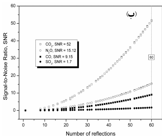
شکل ۱۳. محاسبه وابستگی مقدار SNR به هندسه سلول برای (الف) بیضوی و (ب) دایره‌ای هنگامی که با گازهای مختلف پر شده باشد. پرتو در سلول بیضوی پس از ۱۶۲ بازتاب و در سلول دایره‌ای پس از ۶۰ بازتاب خارج می‌شود.
