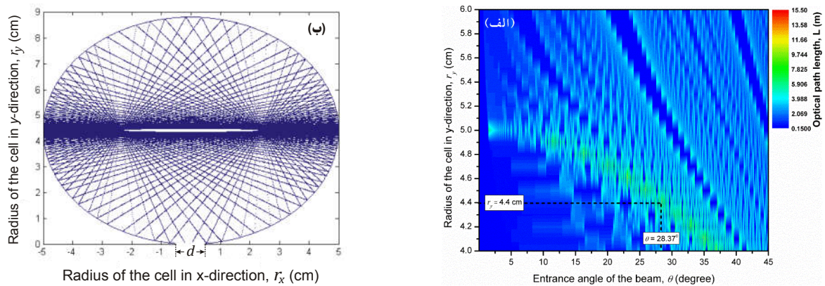
شکل ۵. (رنگی در نسخه الکترونیکی) (الف) بهینه‌سازی طول مسیر پرتو هنگامی که r_x و d به ترتیب در ۵ و یک سانتی‌متر ثابت نگه داشته شده‌اند و r_y و \theta در محدوده نسبتاً مناسبی تغییر کرده‌اند. در این محاسبه مقادیر \theta و r_y به ترتیب با گام‌های یک صدم درجه و یک میلی‌متر تغییر داده شده‌اند. (ب) الگوی مسیر حرکت پرتو در سلول برای مقادیر بهینه به دست آمده در شکل (الف) مقادیر بهینه عبارتند از: r_x = 5 cm، r_y = 4.4 cm و \theta = 28.37^\circ .
