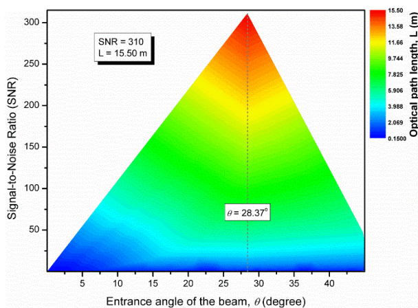
شکل ۱۱. (رنگی در نسخه الکترونیکی) مقدار SNR محاسبه شده از رابطه (۱۶) برای زوایای مختلف ورودی پرتو به سلولی که مشخصات آن در حالت بهینه با توجه به نتایج به دست آمده از شکل ۵ عبارت است از: r_x = 5 cm، r_y = 4.4 cm، d = 1 cm، R_x = 5.088 cm، R_y = 4.451 cm و R = 7.99 . همچنین مشخصات خط گذار (۱۶) عبارتند از: تور P_{CO_2} = 100 و \chi = 10^{-9} ppbv (و 10^{-18} cm -1 /(molecule.cm -1 )) و S_{ij}(\nu) = 3.54 .
