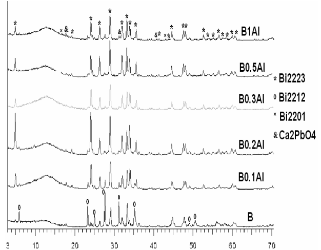
شکل ۱. الگوهای پراش پرتو ایکس نمونه‌های مختلف پس از عملیات کلوخه‌سازی در دمای ۸۱۰ درجه سانتیگراد.
