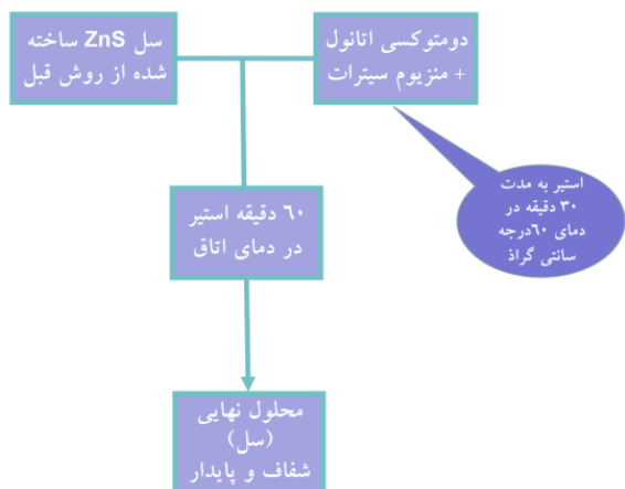
شکل ۲. روش ساخت سل شفاف و پایدار ZnS-Mg.
