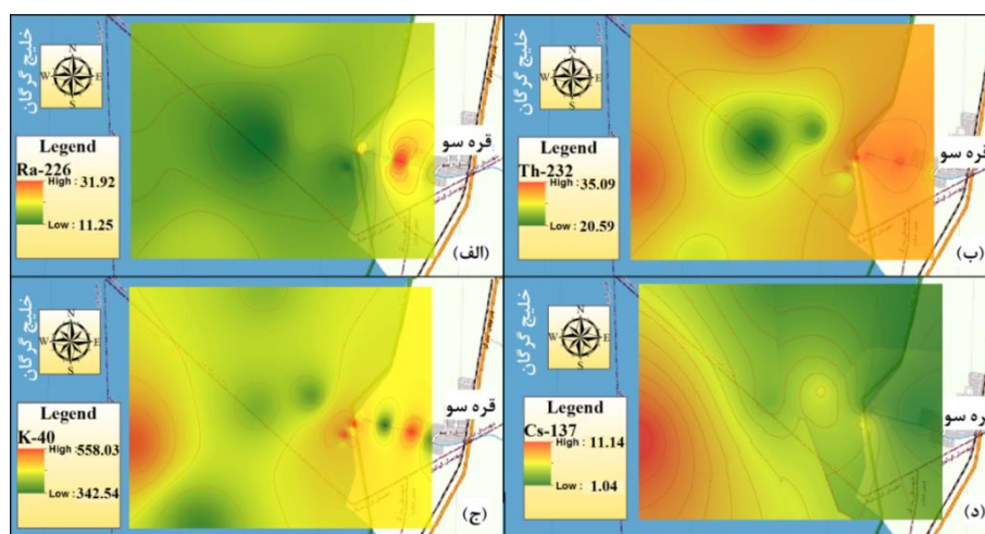
شکل ۸. نمودار هم‌ترازی ^{226}\text{Ra} (الف)، ^{232}\text{Th} (ب)، ^{40}\text{K} (ج) و ^{137}\text{Cs} (د) در ناحیه دهانه رود قره‌سو و قسمت شرقی خلیج گرگان با استفاده از نرم‌افزار GIS.
