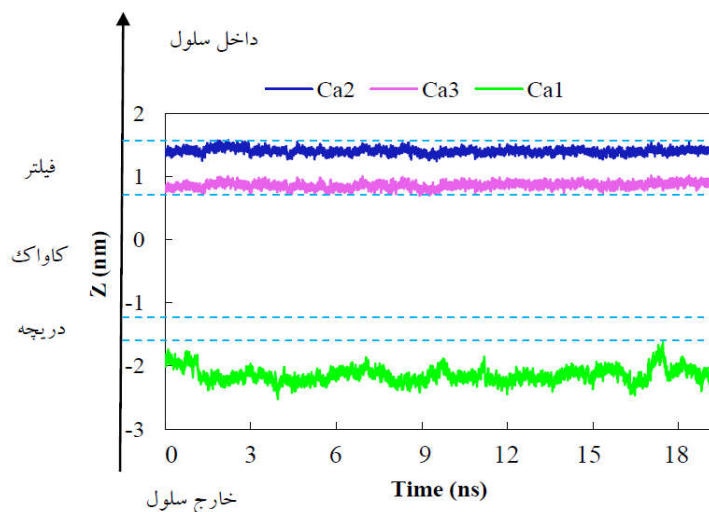
شکل ۳. (رنگی در نسخه الکترونیکی) حرکت یونهای کلسیم (کلسیم ۱ به رنگ سبز، کلسیم ۲: آبی و کلسیم ۳: صورتی) بدون اعمال میدان الکتریکی برای حالت پروتئین فریز شده (بدون غشاء).
