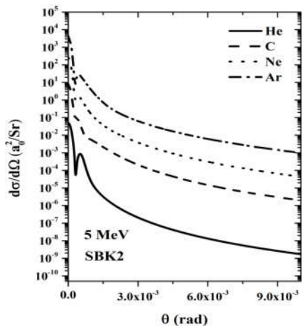
شکل ۱۶. مقایسه نتایج تقریب برینکمن کرامرز ایستای مرتبه دوم برای برخورد پروتون با اتم‌های هلیوم، کربن، نئون و آرگون در انرژی 5 \text{ MeV} .
