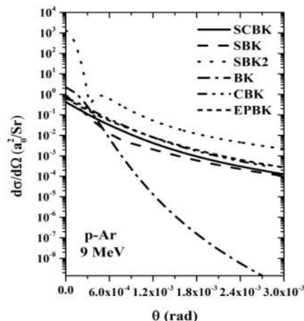
شکل ۱۴. مقایسه سطح مقطع جزئی تقریب‌های برینکمن - کرامرز کولنی پوششی (SCBK)، برینکمن کرامرز ایستا (SBK)، برینکمن کرامرز ایستای مرتبه دوم (SBK2) و برینکمن - کرامرز پتانسیل مؤثر (EPBK) با نتایج تقریب برینکمن - کرامرز مرتبه اول (BK) [۷] و تقریب برینکمن کرامرز کولنی CBK [۷] برای گذار 1s \rightarrow 1s در برخورد پروتون با اتم آرگون در انرژی 9 \text{ MeV} .
