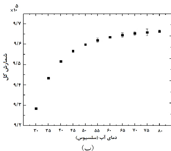
شکل ۳. شمارش (الف) سطح زیر فوتوقله و (ب) سطح زیر کل طیف به ازای تغییرات دمایی آب.
