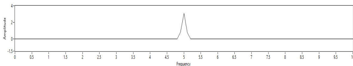
شکل ۷. تبدیل فوریه سیگنال ورودی.
