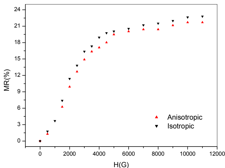
شکل ۴. مغناطومقاومت دو نمونه همسانگرد و ناهمسانگرد \text{La}_{0.78}\text{Sr}_{0.22}\text{MnO}_3 در میدانهای 0-11000 اورستد و دمای 54 درجه کلونین.
