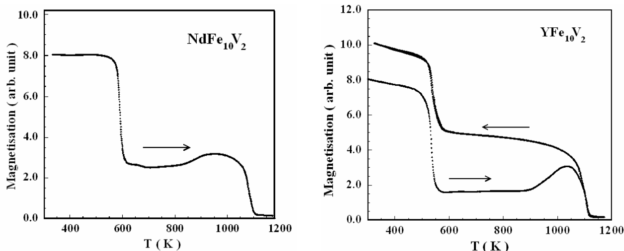
شکل ۳. نتایج اندازه‌گیریهای ترمومغناطیسی که نشان‌دهنده بستگی دمایی مغناطش نمونه‌های YFe_{10}V_2 و NdFe_{10}V_2 در میدان خارجی کوچکتر از 0.1 T و در مقیاس دلخواه هستند. پیکان‌ها جهت افزایش یا کاهش دما را نشان می‌دهند.
