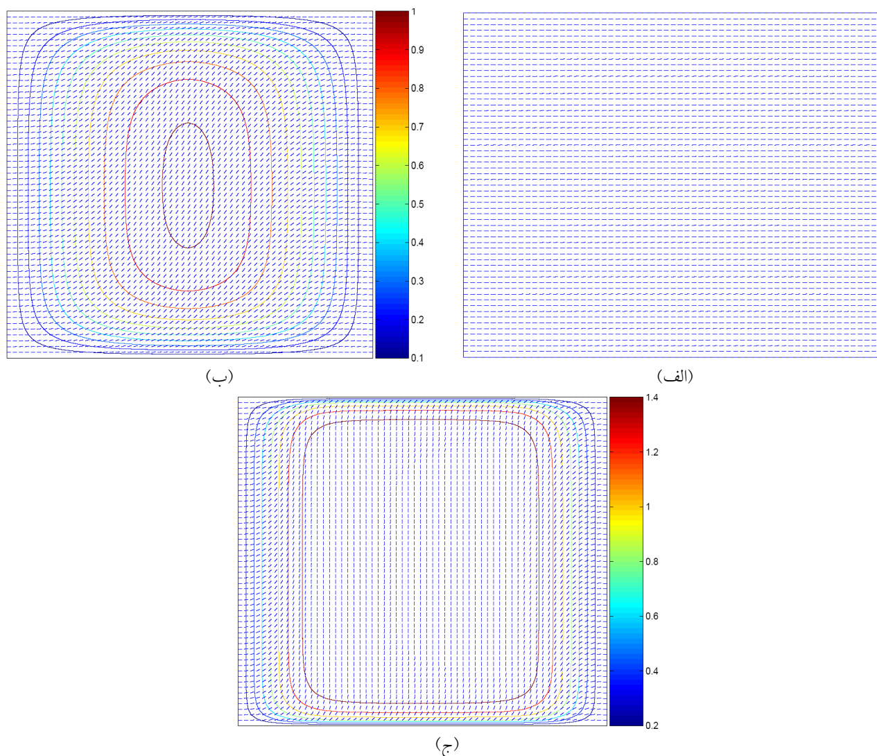
شکل ۶. میدان جهت نما به صورت تابعی از ابعاد برای هندسه چهارگوشی به ازای میدان های مغناطیسی در شرایط (الف) کوچکتر از میدان بحرانی B_c \langle B \rangle ، (ب) بزرگتر از میدان بحرانی B \langle B_c \rangle و (ج) بسیار بزرگتر از میدان بحرانی B \langle B \rangle .
