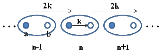
شکل ۶. ساختار شبکه‌ای مدل آیزینگ کوانتمی یک بعدی در میدان مغناطیسی عرضی Jg\sigma_n^x (-1)^n .
