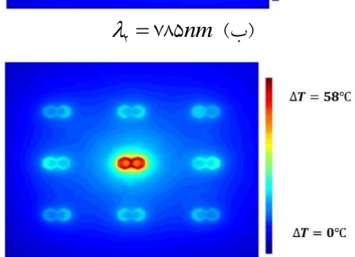
شکل ۴. (الف) توزیع دمایی آرایه نانوذرات دوتایی شش ضلعی در طول موج قله جذب نور با قطبش صفر درجه (۱۲۰۰ نانومتر). (ب) توزیع دمایی آرایه نانوذرات دوتایی شش ضلعی در طول موج ۷۸۵ نانومتر.
