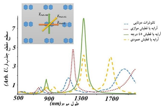
شکل ۵. طیف جذب یک دوتایی شش ضلعی و آرایه‌ای از نانوذرات دوتایی شش ضلعی در قطبش صفر درجه، ۴۵ درجه و ۹۰ درجه.
