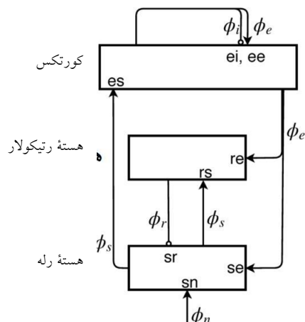
شکل ۱. طرح الگووار ساختار مدل کورتکس-تالاموس مغز که جمعیت نورون‌های کورتکس ( e ) نورون‌های تحریکی، i نورون‌های مهاری) و تالاموس ( r هسته رتیکولار و s هسته رله) را نشان می‌دهد. در اینجا v_{ab} پارامتر وابستگی و قدرت ارتباطات نورون‌های b به a و \phi_a پتانسیل خارجی است [۱۳].
