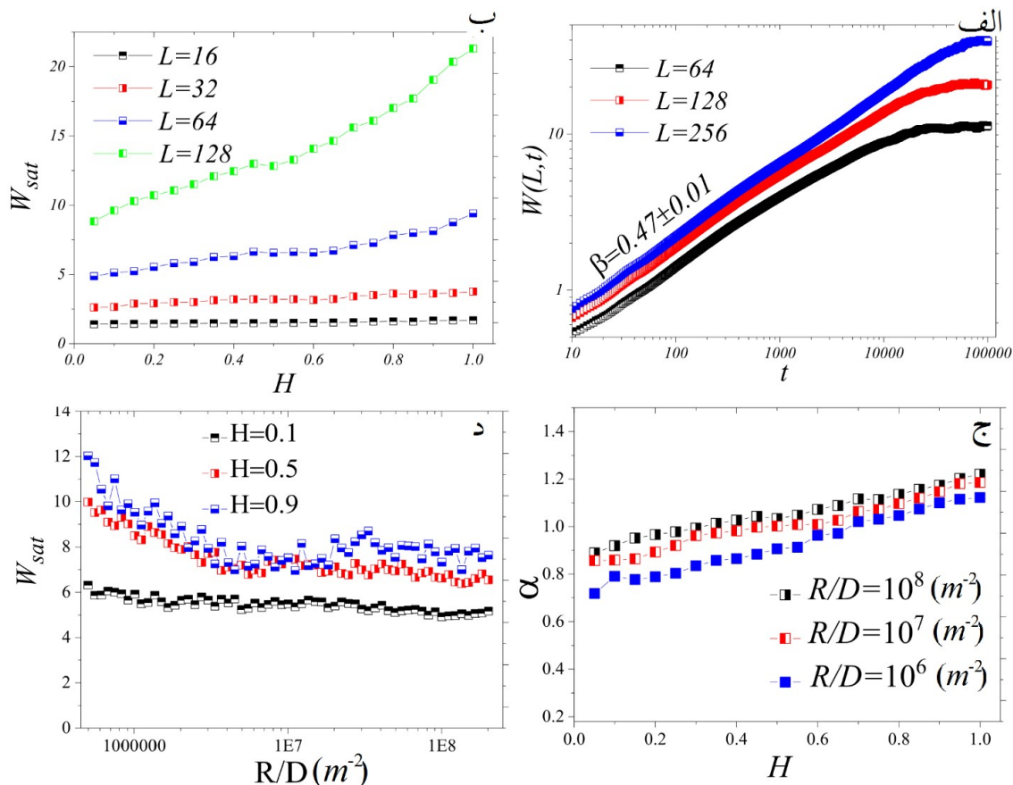
شکل ۵. W(L,t) بر حسب زمان به ازای مقادیر مختلف L (الف)، W_{sat} بر حسب H به ازای مقادیر مختلف L (ب). (ج) \alpha بر حسب H به ازای مقادیر مختلف R/D (د). W_{sat} بر حسب R/D به ازای مقادیر مختلف H .
