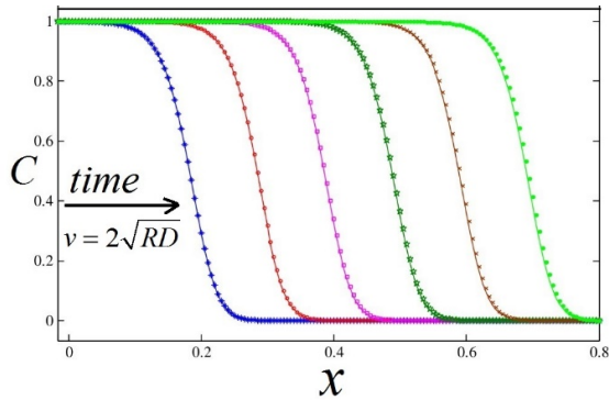
شکل ۱. جبهه موج و حرکت آن در معادله فیشر یک بعدی.
