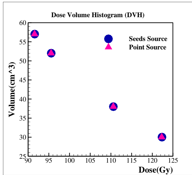
شکل ۸. مقادیر دز جذبی پرتو بافت سرطانی در طرح درمانی اول. همزمان چشمه‌های نقطه‌ای و دانه‌ای خطی در یک نمودار رسم شده‌اند.
