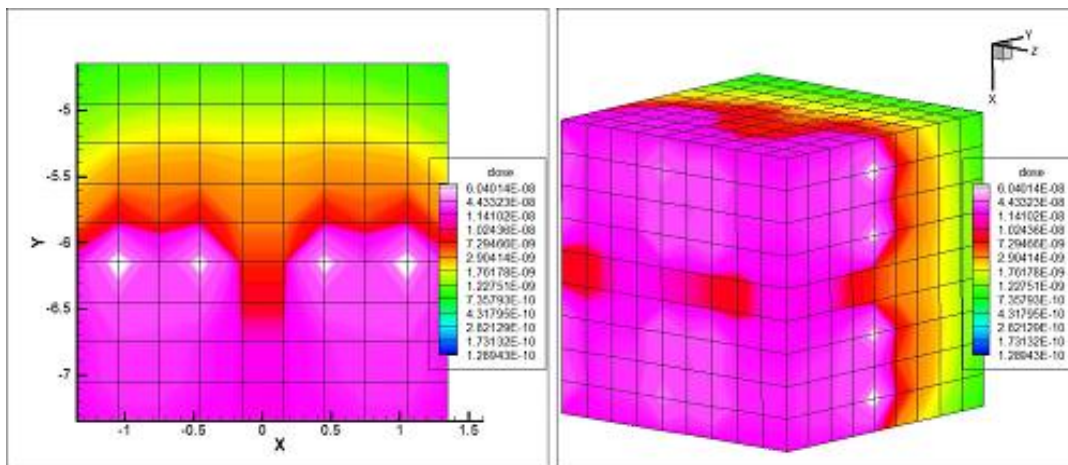
شکل ۹. منحنی هم دز تجمعی پروستاتی با حجم ۳۰/۰۲ سانتی مترمکعب با جایگذاری ۷۶ چشمه دانه‌ای خطی طبق طرح درمانی.
