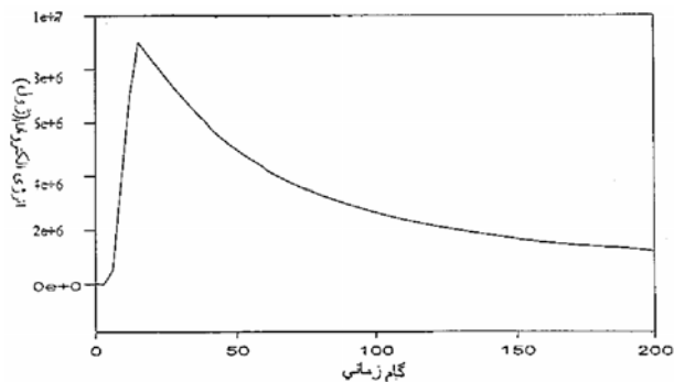
شکل ۹. نمودار انرژی الکترونی گسیل شده از سوخت در گام‌های زمانی ۰/۱ پیکوثانیه
