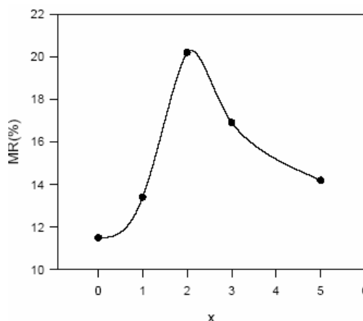
شکل ۱۶. نمودار MR برای نمونه‌های LSMO/xTiO 4 در میدان ۸۰۰۰ اورستد و دمای ۷۷ کلوین.
