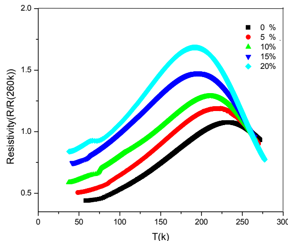
شکل ۲۶. تغییرات مقاومت الکتریکی نمونه‌های La_{0.8}Sr_{0.2}MnO_3 / x LaMnO_3 با دما.
