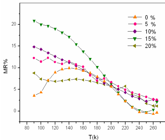
شکل ۲۷. تغییرات مغناطومقاومت نمونه‌های La_{0.8}Sr_{0.2}MnO_3 / x LaMnO_3 با دما.
