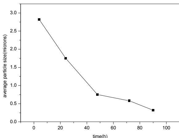
شکل ۲۸. طرح واره‌ای از توزیع اندازه ذرات La_{0.8}Sr_{0.2}MnO_3 که در مدت زمان‌های مختلف آسیاب شده‌اند.
