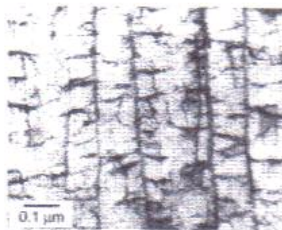
شکل (۳-الف). سیلیکان متخلخل ساخته شده از سیلیکان نوع n. شدت جریان 10 \text{ mA/cm}^2 ، غلظت الکترولیت ۴۹٪ (HE)، جهت جریان از پایین صفحه به سمت بالاست [۳].
