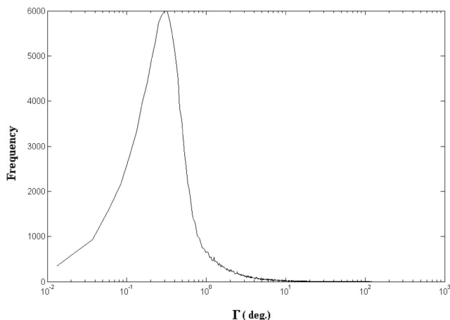
شکل ۷. تابع توزیع زاویه بین جهت ذره اولیه و جهت میانگین ذرات ثانویه.
