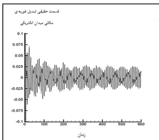
شکل ۴. نمودار قسمت حقیقی تبدیل فوری مکانی میدان الکتریکی بر حسب زمان.
