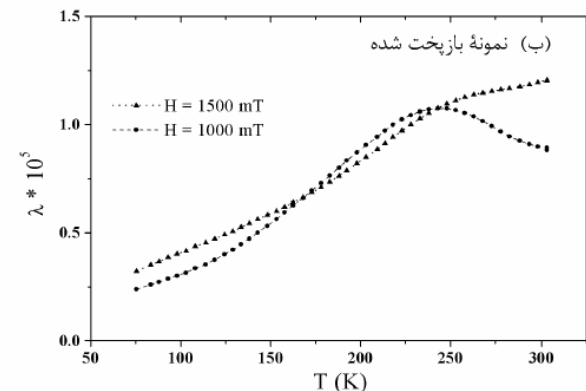
شکل ۸. وابستگی دمایی مغناطوتنگش نمونه‌های نانوکامپوزیتی به همبسته با پلیمر \text{Nd}_2\text{Fe}_{14}\text{B}_{17.5}\text{B}_{17.5} ، (الف) نمونه اصلی، (ب) نمونه بازپخت شده.
