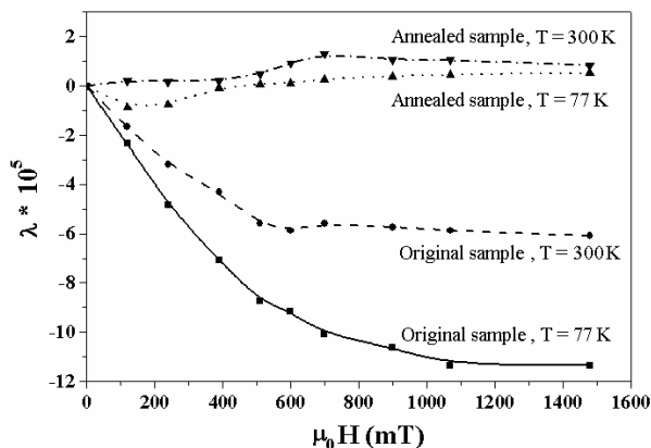
شکل ۷. منحنیهای همدمای مغناطوستنگش بر حسب میدان خارجی در نمونه نانوکامپوزیتی به هم بسته با پلیمر \text{Nd}_7\text{Fe}_{14}\text{B}_{18/5} پس از گرمادهی در دمای 700^\circ\text{C} به مدت ۱۰ دقیقه.
