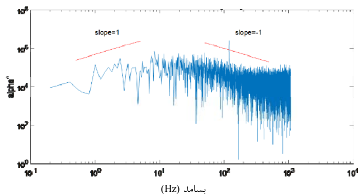
شکل ۸. (رنگی در نسخه الکترونیکی) نمودار تابع \alpha'' بر حسب بسامد.
