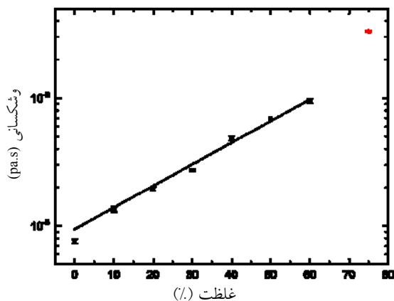
شکل ۴. (رنگی در نسخه الکترونیکی) نمودار نشان دهنده تغییرات وشکسانی با غلظت مخلوط آب و گلیسرین است. که نقاط به ترتیب ۰٪ محلول آب و مخلوط آب و گلیسرین ۱۰٪، ۲۰٪، ۳۰٪، ۴۰٪، ۵۰٪، ۶۰٪ و ۷۵٪ است.
