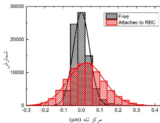
شکل ۶. (رنگی در نسخه الکترونیکی) نمودار فراوانی مکان ذره نسبت به مرکز تله در حالت آزاد (سیاه) و حالت متصل به گلبول (قرمز).
