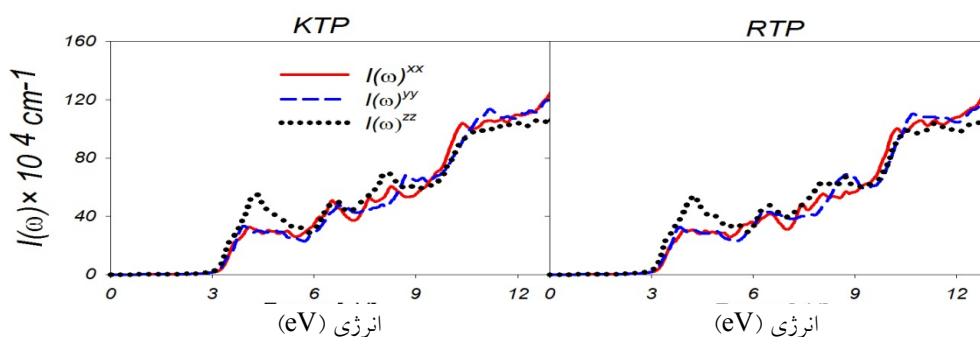
شکل ۸. (رنگی در نسخه الکترونیکی) نمودار طیف جذب KTP و RTP.
