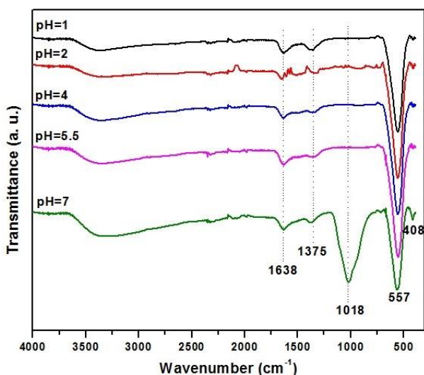
شکل ۶. طیف‌های تبدیل فوریه فروسرخ پودرهای سنتز شده در مقادیر مختلف pH در حضور اندازه ثابت نمک.
