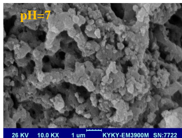
شکل ۱۰. ریزساختارهای نمونه‌های سنتز شده در مقادیر مختلف pH در حضور مقدار ثابت نمک.
