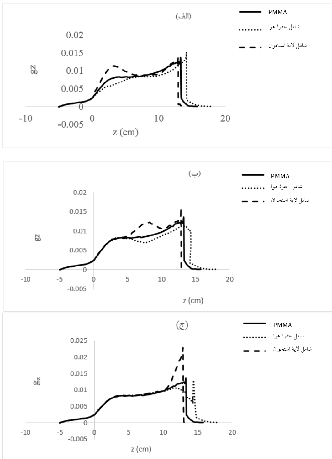
شکل ۶. توزیع مکانی گسیل گامای آنی یک پروتون در واحد زمان ناشی از تبدیل PGT شبیه‌سازی شده، برای هدف همگن PMMA و اهداف PMMA با لایه استخوان یا حفره هوا در مکان‌های ۲۰ mm، ۷۰ mm و در قله براگ (که لایه استخوان در مکان ۱۲۰ mm و حفره هوا در مکان ۱۳۰ mm) است به ترتیب در (الف)، (ب) و (ج) مورد مقایسه قرار گرفته‌اند.
