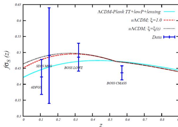
شکل ۷. نمودار پارامتر f\sigma_8 بر حسب z برای مدل \Lambda CDM با بهترین برازش داده‌های Planck2015 TT + low P + lensing و \ddot{u} \Lambda CDM با بهترین برازش داده‌های Planck 2015 + R16 + BAO برای \ddot{u} \Lambda CDM دو حالت \xi = 1 و \xi = \xi(z) در نظر گرفته شده است [۷].
