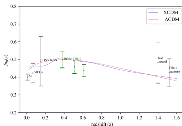
شکل ۸. نمودار پارامتر f\sigma_8 در دو مدل \Lambda CDM و XCDM. اندازه‌گیری‌های رصدی از منابع [۱۱]، [۳۱]، [۳۲]، [۳۳]، [۳۴] و [۳۵] هستند.
