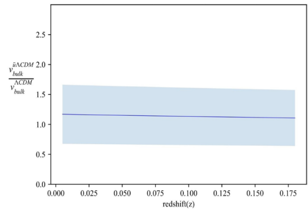
شکل ۳. نسبت متوسط جریان توده پیش‌بینی شده در مدل \Lambda CDM به متوسط جریان توده در \Lambda CDM.
