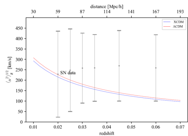
شکل ۴. نمودار جذر میانگین مربعی سرعت در دو مدل استاندارد و XCDM. داده‌های ابرنواخترها مربوط به کاتالوگ Union 2 هستند. [۷] داده‌های ابرنواخترها جریان توده‌ای در حدود \frac{260 \text{ km}}{s} را تا انتقال به سرخ z = 0.06 نشان می‌دهند.
