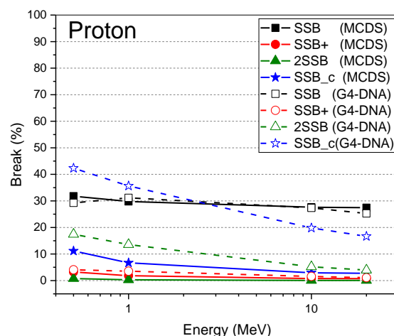
شکل ۵. مقایسه احتمال شکست‌های تک‌رشته‌ای پروتوهای پروتون در DNA سلول، محاسبه شده در این پژوهش با کد MCDS (خطوط پررنگ و اشکال توپر) در مقایسه با نتایج کد Geant4-DNA (خطوط نقطه‌چین و اشکال توخالی) [۱۲].
