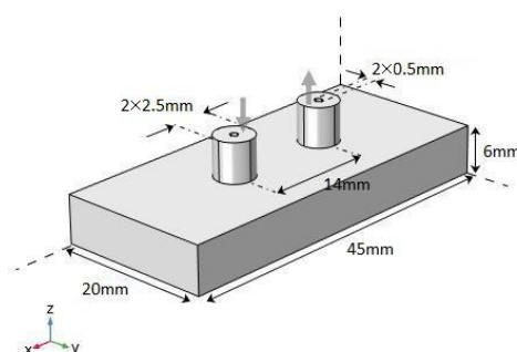
شکل ۱. یک کاواک موج میکرو مکعب مستطیلی با ابعاد (a, b, d) = (45, 20, 6) mm به ترتیب در راستاهای x ، y و z . شعاع داخلی، شعاع خارجی و فاصله جدایی میان دو درگاه کاواک به ترتیب عبارتند از 0.5 mm، 2/5 mm و 14 mm.
