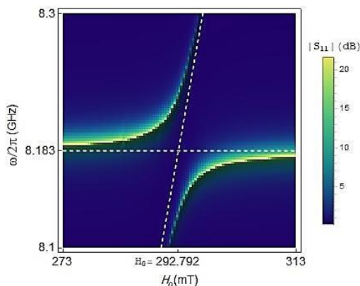
شکل ۶. نمودار اندازه طیف بازتابی موج میکرو |S_{11}| بر حسب بسامد و میدان مغناطیسی خارجی برای ویژه مد TM_{110} در حضور یک کره مغناطیسی با شعاع 0.5 \text{ mm} ؛ خطچین افقی و مایل به ترتیب مد کاواک \omega_c و مد کره مغناطیسی \omega_m را مشخص می کنند.
