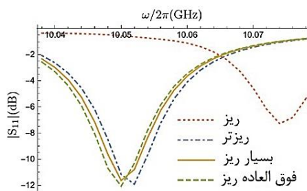
شکل ۵. نمودار اندازه طیف بازتابی موج میکرو |S_{11}| در حوالی یک بسامد تشدید سامانه جفت شده کاواک موج میکرو و کره مغناطیسی به ازای اندازه‌های مختلف شبکه‌بندی کره مغناطیسی.
