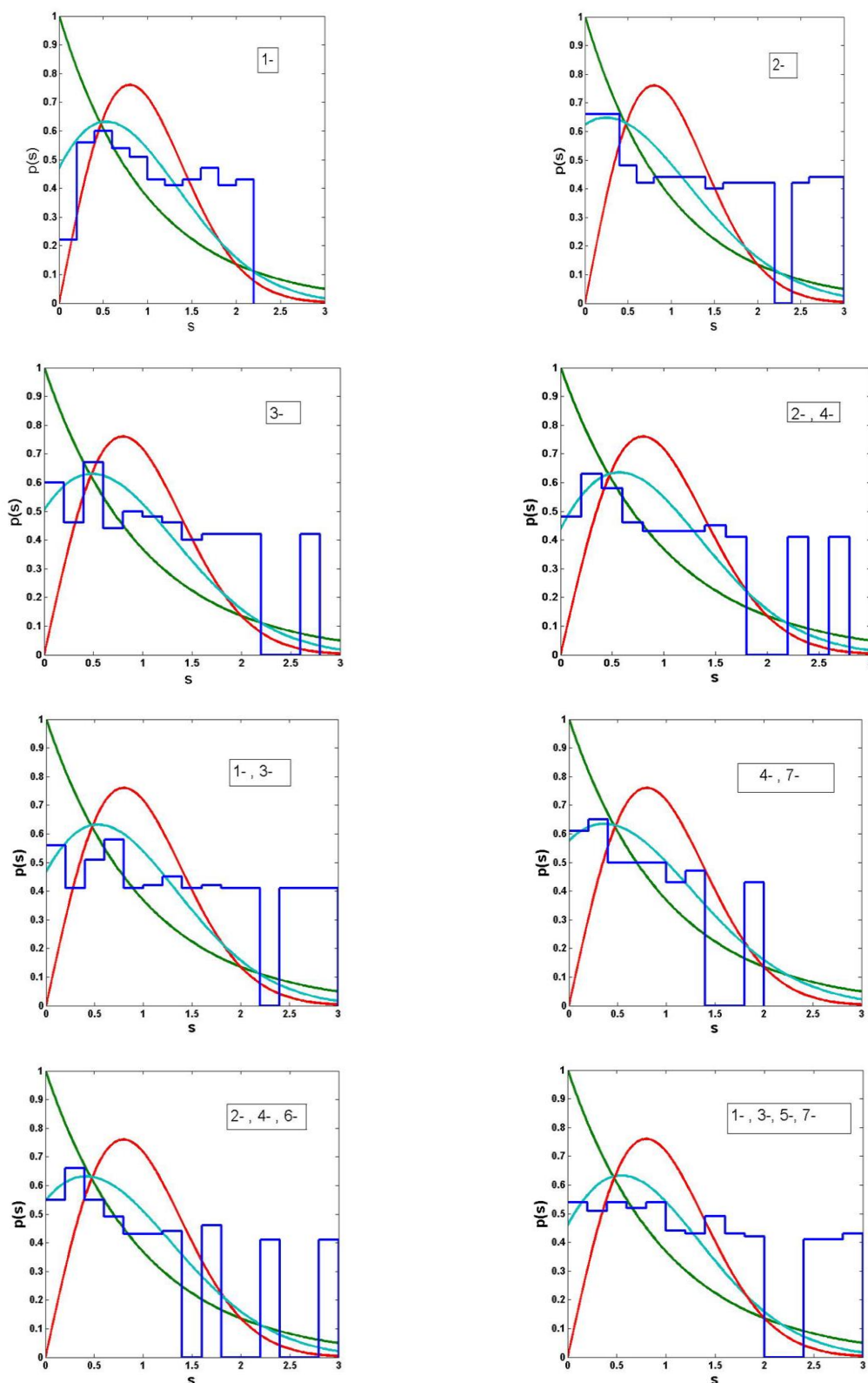
شکل ۱. توزیع نزدیک‌ترین فاصله بین ترازهای (NNSD) برای ترازهای مختلف انتخابی با پارامتر منفی. در تمام شکل‌ها، محور افقی کمیت s فاصله نسبی بین ترازهای مورد مطالعه بعد از فرایند واپیچش و محور عمودی، P(s) احتمال هر بازه انتخابی را نشان می‌دهد. همچنین ستون‌های آبی رنگ، هیستوگرام داده‌های تجربی، نمودار سبز، تابع توزیع پواسونی، نموداری، تابع توزیع گوسی و نمودار قرمز رنگ، تابع توزیع بری - روبینیک را توصیف می‌کند.
