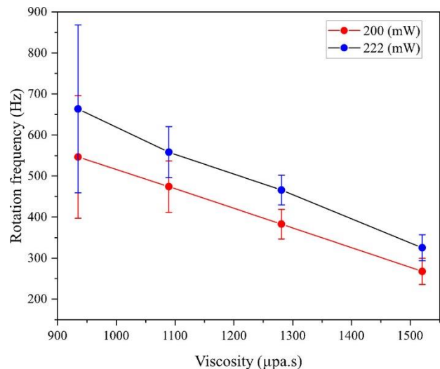
شکل ۶. اثر وشکسانی محیط بر روی سرعت چرخش ذره. فرکانس چرخش بر حسب وشکسانی مخلوط آب و گلیسرین با نسبت‌های مختلف، برای دو توان لیزر مختلف ۲۰۰ mW و ۲۲۲ mW قبل از عدسی شیئی رسم شده است.
