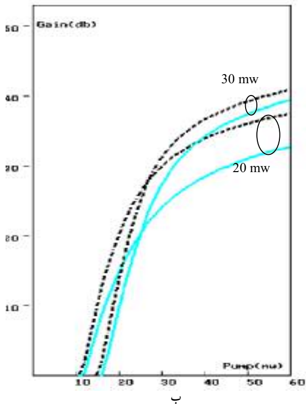
شکل ۷. منحنی بهره تقویت برحسب توان پمپ برای فیبر رایج تک مدی در طول موج پمپ ۰/۹۸ میکرومتر، شکل (الف): برای طولهای بهینه در توانهای پمپ ۱۰ و ۱۵ میلی وات. شکل (ب): برای طولهای بهینه در توانهای پمپ ۲۰ و ۳۰ میلی وات.
