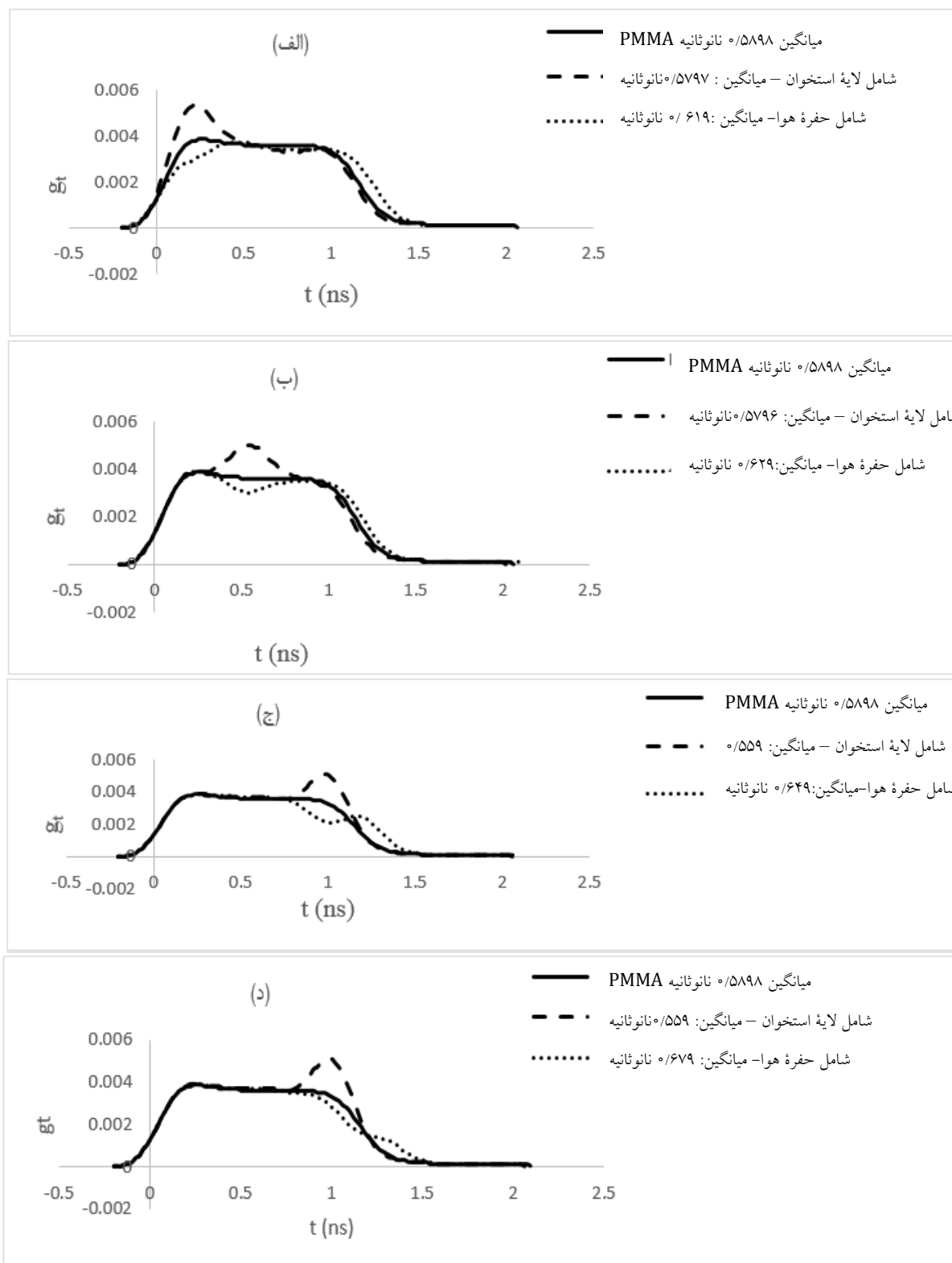
شکل ۵. طیف PGT یک پروتون در واحد زمان برای هدف همگن PMMA و اهداف PMMA با لایه استخوان یا حفره هوا در مکان (الف) ۲۰ mm، (ب) ۷۰ mm، (ج) ۱۲۰ mm و (د) محل قلّه براگ.
