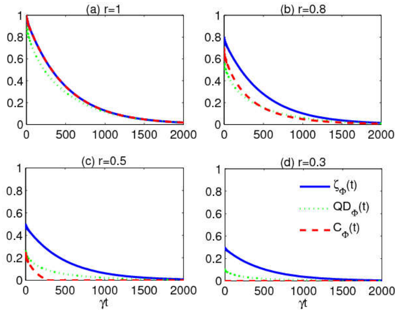
شکل ۴. (رنگی در نسخه الکترونیکی) دینامیک همدوسی (نمودار پر آبی)، ناسازگاری کوانتومی (نمودار نقطه چین سبز)، درهم‌تندگی (نمودار خط چین قرمز) به ازای مقادیر مختلف شاخص خلوص r : (a) r=1 ، (b) r=0.8 ، (c) r=0.5 و (d) r=0.3 و حالت اولیه \rho_{\Phi}(0) . سایر پارامترها عبارتند از: \lambda=0.05\gamma ، \beta=0.5 \times 10^{-9} ، \omega_0=1.53 \times 10^9 ، C_1=C_2=1/\sqrt{2} و \Delta=0 .
