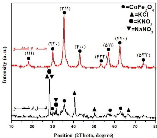
شکل ۱. الگوی پراش پرتو ایکس پودرهای سنتز شده در نسبت مولی KCl به مجموع نیترات‌های فلزی به اندازه دو سوم و pH محلول اولیه یک.
