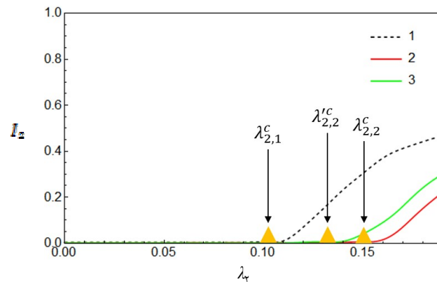
شکل ۱۲. (رنگی در نسخه الکترونیکی) جمعیت افراد مبتلا به بیماری ۲ بر حسب \lambda_1 ، در حالت رقابت دو بیماری. هر دو شبکه اردوش-رنیی هستند با \langle k \rangle = 7 و \langle I \rangle = 8 . آستانه اولیه انتشار با \lambda_{2,1}^c و آستانه ثانویه در حالتی که بیماری ۲ در ابتدای فرایند انتشار وارد شده با \lambda_{2,2}^c و در حالتی که در انتهای فرایند انتشار وارد شد با \lambda_{2,2}'^c نشان داده شده است.
