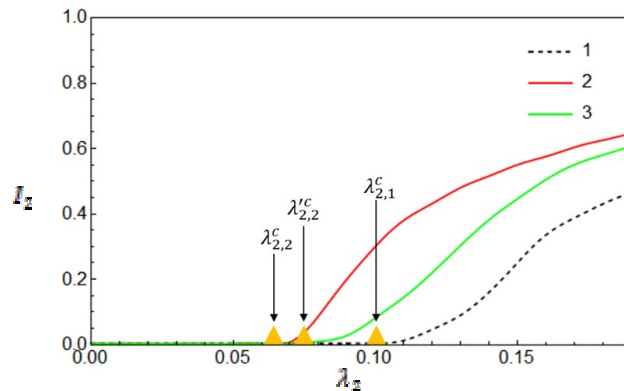
شکل ۱۱. (رنگی در نسخه الکترونیکی) جمعیت افراد مبتلا به بیماری ۲ بر حسب \lambda_2 ، در حالت همکاری دو بیماری. هر دو شبکه اردوش-رنیی هستند با \langle k \rangle = 7 و \langle I \rangle = 8 . آستانه اولیه انتشار با \lambda_{2,1}^c و آستانه ثانویه در حالتی که بیماری ۲ در ابتدای فرایند انتشار وارد شده با \lambda_{2,2}^c و در حالتی که در انتهای فرایند انتشار وارد شد با \lambda_{2,2}'^c نشان داده شده است.
