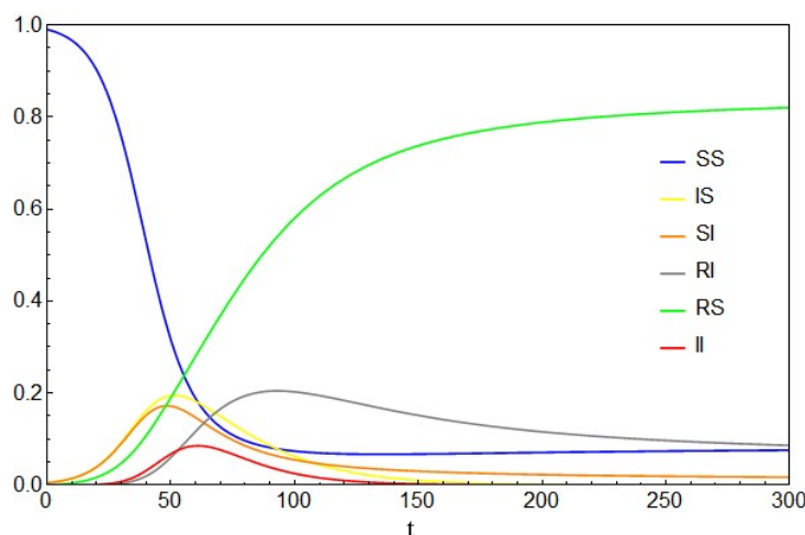
شکل ۴. (رنگی در نسخه الکترونیکی) تحول مدل SIR-SIS بر حسب زمان در حالت رقابت دو بیماری. متوسط درجهٔ رئوس در هر دو شبکهٔ منظم k=l=8 است. پارامترهای دینامیکی برابرند با: \lambda_1 = \lambda_2 = 0.02 ، \gamma_1 = \mu_2 = 0.05 ، \beta_1^a = \beta_1^b = \beta_2^a = \beta_2^b = 0.18 ، \phi_2^a = \phi_2^b = 0.06 و \eta_1 = \eta_2 = \zeta_2 = 1/3 .
