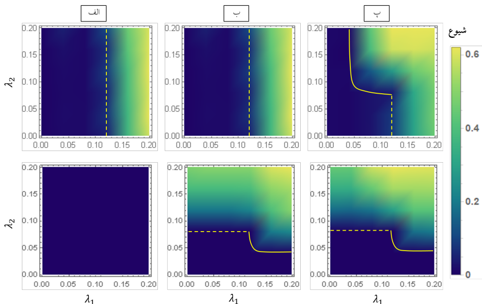
شکل ۵. (رنگی در نسخه الکترونیکی) نمودار فاز مدل در حالت همکاری دو بیماری بر روی دو شبکه اردوش-رنی با N_1 = N_2 = 5000 و \langle l \rangle = 8, k = 7 . سطر اول میزان شیوع بیماری ۱ و سطر دوم میزان شیوع بیماری ۲ را در فضای (\lambda_1, \lambda_2) نشان می‌دهند. در ستون (الف) بذر بیماری ۱ ( IS=0.005 )، در ستون (ب) بذر بیماری ۲ ( SI=0.005 ) و در ستون (پ) مجدداً بذر بیماری ۱ ( IS=0.005 )، در حالت پایا به سیستم اضافه شده است. پارامترهای دینامیکی برابرند با: \phi_1^a = \phi_2^b = 1/2, \zeta_2 = 0.8, \gamma_1 = \mu_2 = 0.75, \beta_1^a = \beta_1^b = \beta_2^a = \beta_2^b = 1/3 و \eta_1 = \eta_2 = 0.8 .
